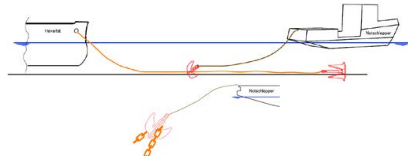
Prinzipskizze Notschleppdragen
